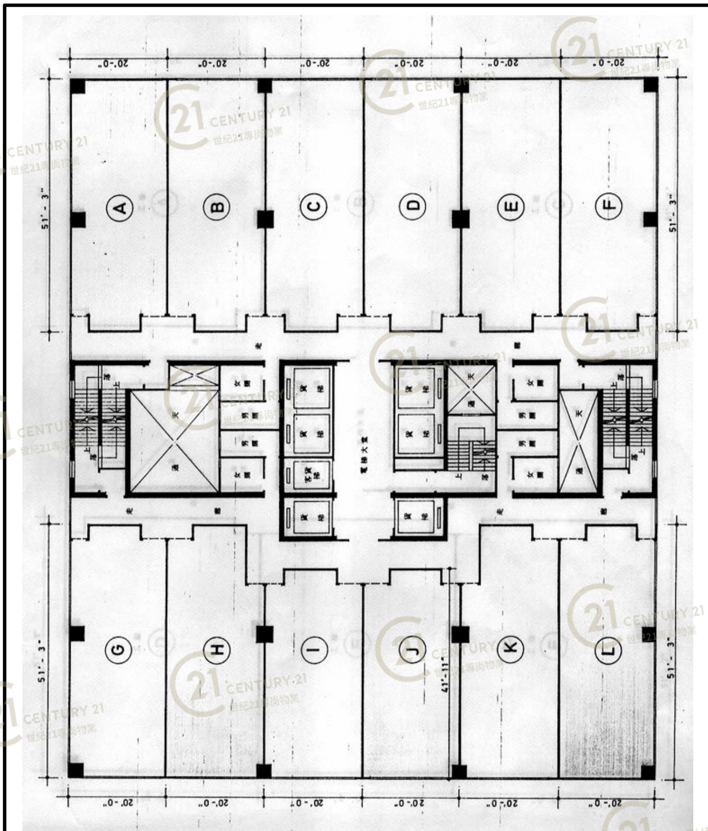
三樓至九樓平面圖
